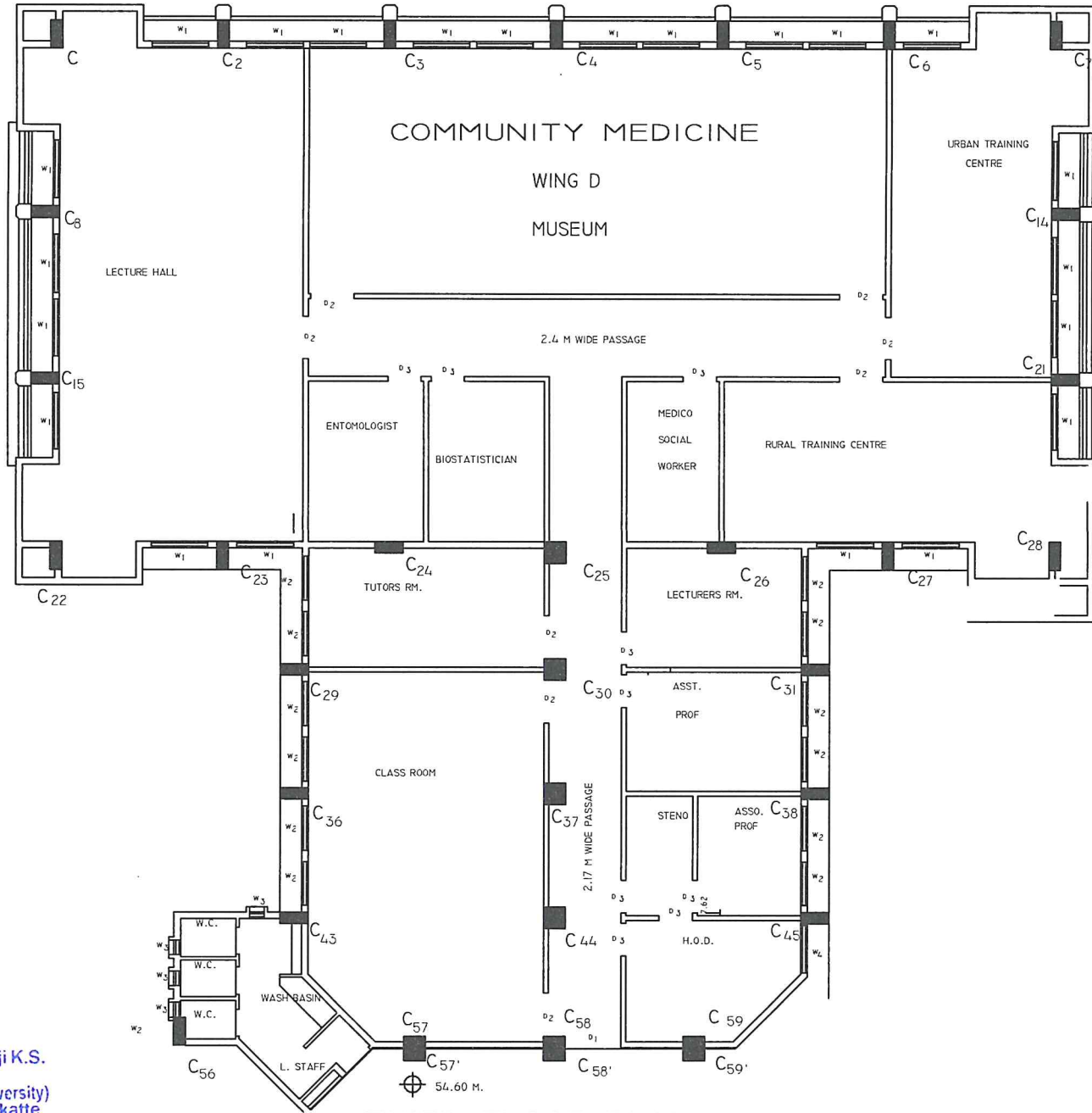
THIRD FLOOR PLAN 712.22 SOM Page 36 of 100
